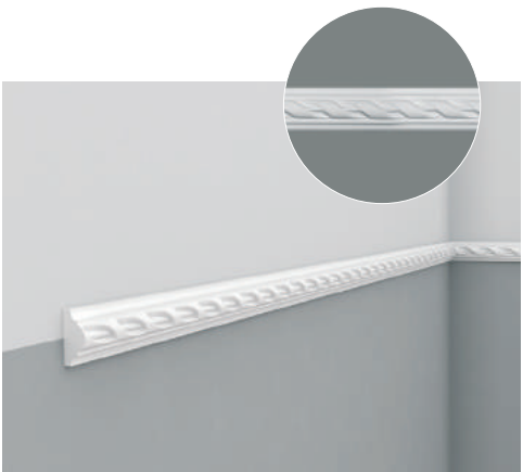
MDC252 240 x 5,1 x 1,9 cm | Flex 235 cm PRESTIGE Flex
